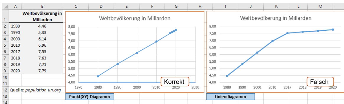
Korrekte Datendarstellung (Punkt (XY)-Diagramm) und falsche Darstellung (Liniendiagramm)
